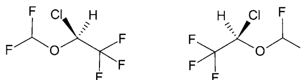
Obr. 3. Štruktúry izomérov izofluranu (S)-izoflurán (R)-izoflurán
