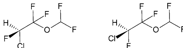
Obr. 1. Enantioméry enfluranu (S)-(+)-enflurán (R)-(-)-enflurán
