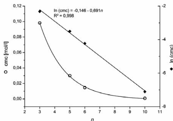
Graf 2. Závislosť hodnôt cmc a \ln(cmc) od počtu atómov uhlíka n v hydrofóbnom reťazci študovaných pyrolidínoetylerov m -alkoxysubstituovanej kyseliny fenylykarbámovej
