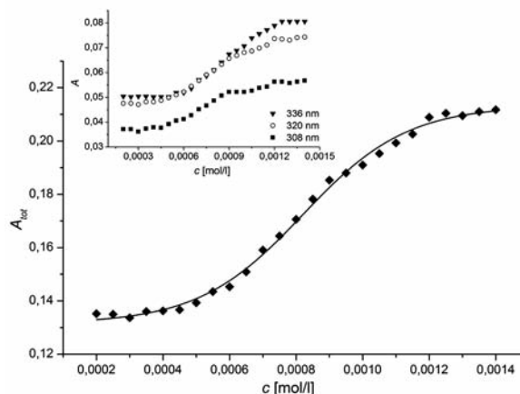
Graf 1. Závislosť súčtu absorbancií hlavných pyrénových pík ( A_{tot} ) od koncentrácie ( c ) látky XXIX Z vo vodnom prostredí pri 25 °C
