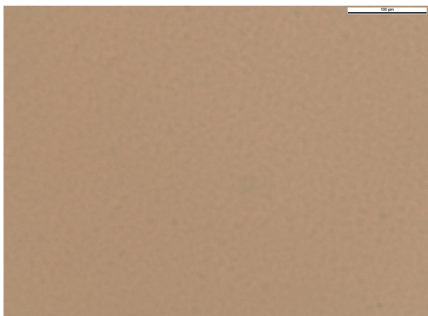
Obr. 3. Lidokainový emulgel s 5 % lidokainu, 0,6 % thymolu bez přísady trometamolu (90. den od přípravy, zvětšení 400x)
