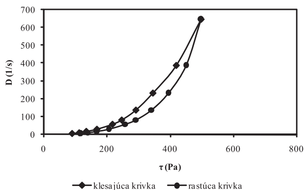
Graf 3. Toková krivka hydrogélů s obsahom: 2,5 % CHIT (typu B) + 5 % SAL + 5 % GLY
