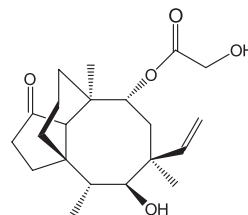
Obr. 24. Pleuromutilin – inhibitor proteosyntézy
