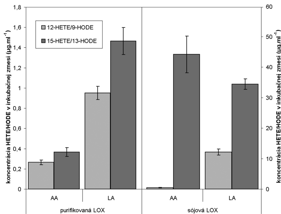
Obr. 6. Porovnanie spektra produktov purifikovanej a sójovej LOX inkubovaných s AA a LA
