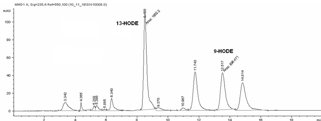
Obr. 5. SP-HPLC záznam produktov inkubácie vzorky s kyselinou linolovou Rt = 8,498: 13-HODE; Rt = 13,517: 9-HODE
