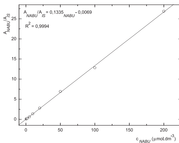
Obr. 6. Závislost odezvy standardních roztoků nabumetonu na koncentraci (kolona Supelcosil LC-18 15cm \times 4,6 mm 5 \mu\text{m} ; ACN : 0,1% TFA 50 : 50 0,3 ml.min -1 ; nástřik 30 \mu\text{l} , MS m/z 171, m/z 185)
