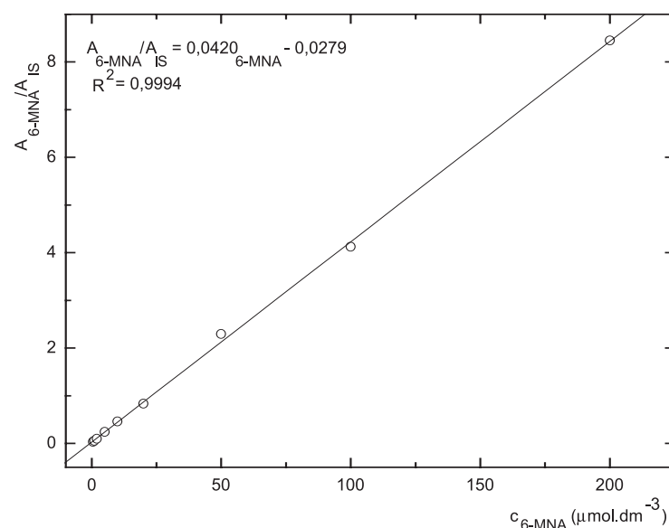
Obr. 7. Závislost odezvy standardních roztoků 6-MNA na koncentraci (kolona Supelcosil LC-18 15cm \times 4,6 mm 5 \mu\text{m} ; ACN : 0,1% TFA 50 : 50 0,3 ml.min -1 ; nástřik 30 \mu\text{l} , MS m/z 171, m/z 185)
