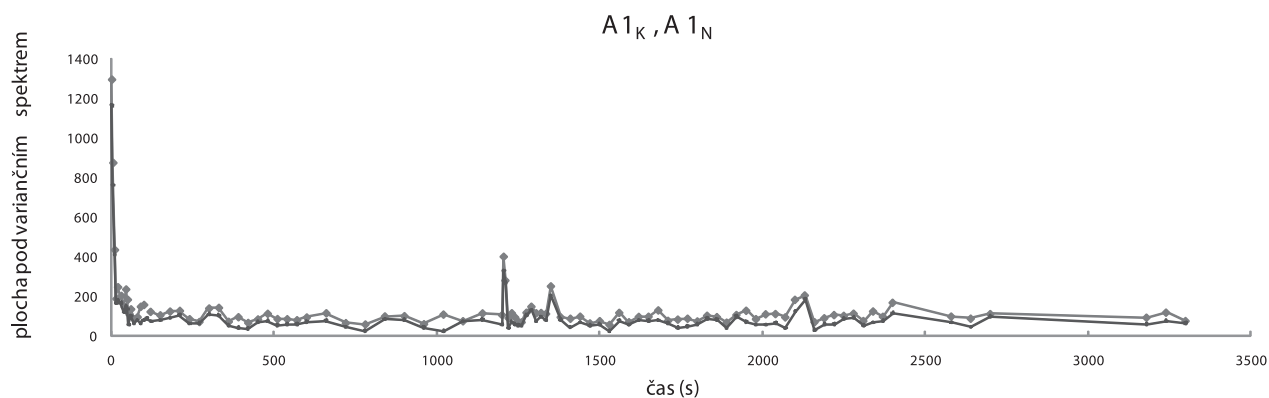
Obr. 8. Znáznornění průběhu homogenizace vzorku V2S100. (◆) data metody A1_N (odečet nekorigovaných ploch); (■) data metody A1_K (odečet korigovaných ploch)
