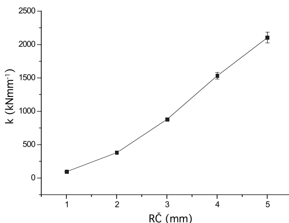
Obr. 5. Vliv rychlosti čelisti RČ na rychlostní konstantu drtícího procesu k
