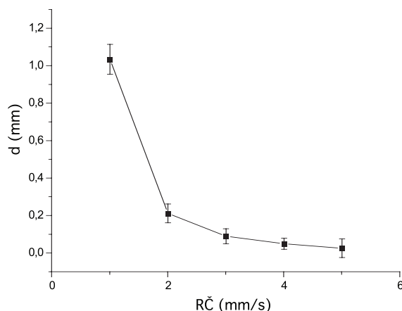
Obr. 4. Vliv rychlosti čelisti RČ na dráhu drcení d
