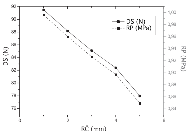
Obr. 3. Vliv rychlosti čelisti RČ na drtící sílu DS a radiální pevnost RP tablet
