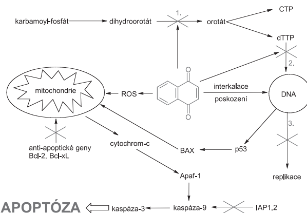
Obr. 3. Mechanismus účinku naftochinonů zahrnuje inhibici dihydroorotát dehydrogenasy (1) a inkorporaci thymidinu do DNA (2), dále inhibici některých enzymů replikace DNA – topoizomerasy (3). Naftochinony jsou rovněž schopny generovat reaktivní formy kyslíku (ROS). Ve schématu je vyznačena down-regulace některých antiapoptických genů (rodina Bcl genů, IAP genů).
