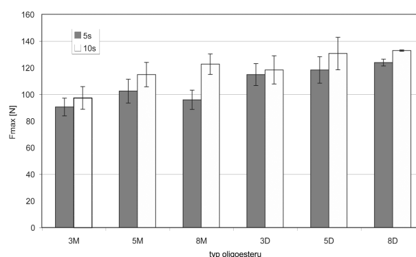
Obr. 2. Vliv doby kontaktu adheziva s podkladem na velikost adhezivní síly – kontaktní síla 20 N, rychlost odtržení vzorku od podkladu 100 mm/min F_{max} (N) – průměrná maximální síla (5 měření) při odtržení adheziva od substrátu, 3M ... 8D – oligoestery větvené 3, 5 nebo 8% mannitolu (M) nebo dipentaerythritolu (D) 5 s, 10 s – doba kontaktu adheziva s podkladem
