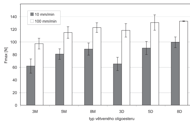
Obr. 3. Vliv rychlosti odtržení adheziva od podkladu na velikost adhezivní síly – kontaktní síla 20 N, doba kontaktu 10 s F_{max} (N) – průměrná maximální síla (5 měření) při odtržení adheziva od substrátu, 3M ... 8D – oligoestery větvené 3, 5 nebo 8% mannitolu (M) nebo dipentaerythritolu (D), 10 mm/min, 100 mm/min – rychlost odtržení adheziva od podkladu
