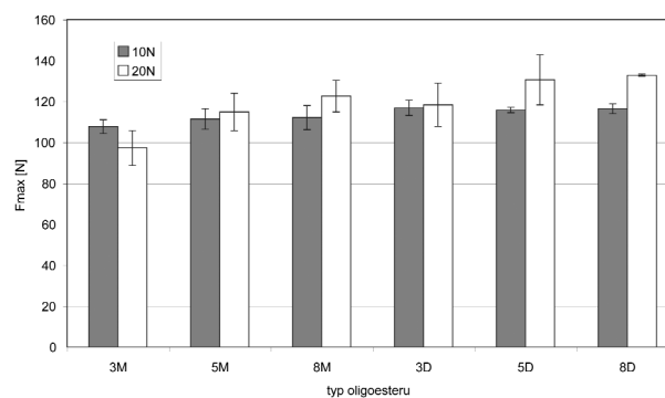
Obr. 1. Vliv kontaktní síly na velikost adhezivní síly – doba kontaktu 10 s, rychlost odtržení vzorku od podkladu 100 mm/min F_{max} (N) – průměrná maximální síla (5 měření) při odtržení adheziva od substrátu, 3M ... 8D – oligoestery větvené 3, 5 nebo 8% mannitolu (M) nebo dipentaerythritolu (D), 10 N, 20 N – kontaktní síla
