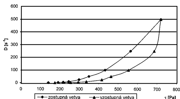
Obr. 2. Toková krivka 1,5% hydrogélů Carbopolu® 980 D – rýchlostný spád, \tau – tangenciálne napätie
