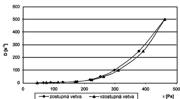
Obr. 1. Toková krivka 0,5% hydrogélů Carbopolu® 980 D – rýchlostný spád, \tau – tangenciálne napätie
