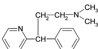
Obr. 1. Vzorec feniramínu
