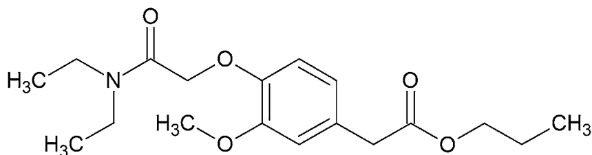
Obr. 9. Chemická štruktúra propanididu
