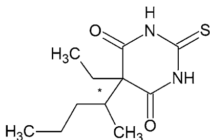
Obr. 1. Chemická štruktúra tiopentalu
