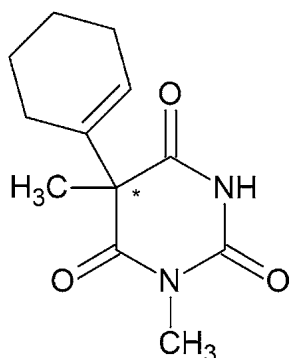
Obr. 3. Chemická štruktúra hexobarbitalu
