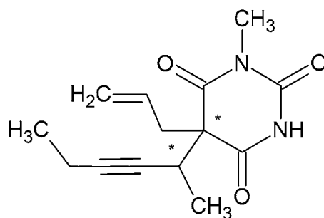
Obr. 2. Chemická štruktúra metohexitalu
